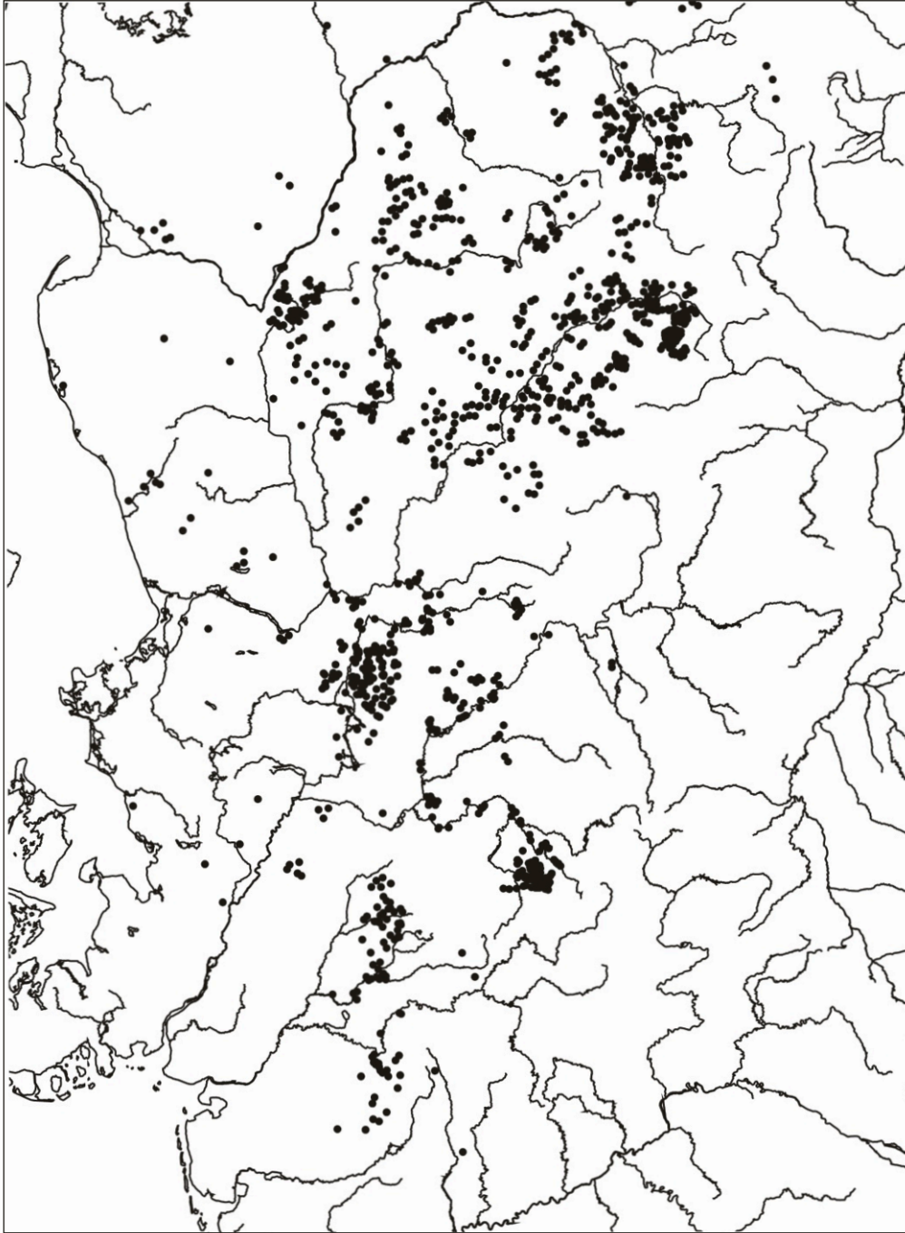
Fig. 1. Răspândirea ceramicii lucrate la roată din perioada romană-târzie și a migrațiilor. Prezentare schematică (lista 1).
